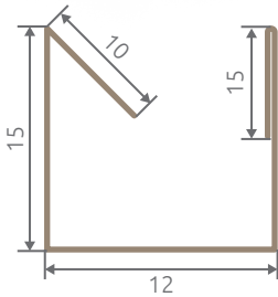
Alsó oromszegés
