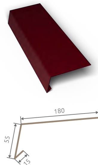
Cseppentő
