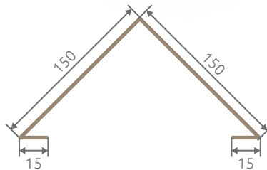
Falszegés (felső)
